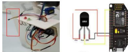
Gambar 4. Rangkaian sensor Suhu ke NodeMcu esp8266
